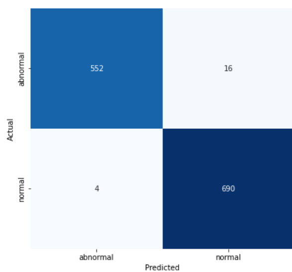
Xception
