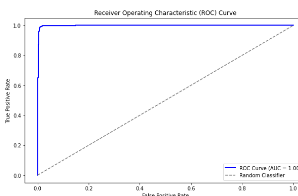
MobileNetV2
