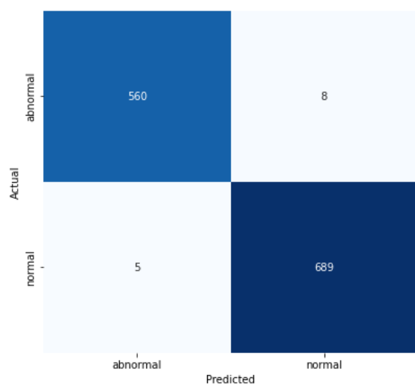
MobileNetV2
